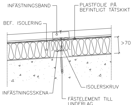
Figur 6.4 Infästning med skena.
