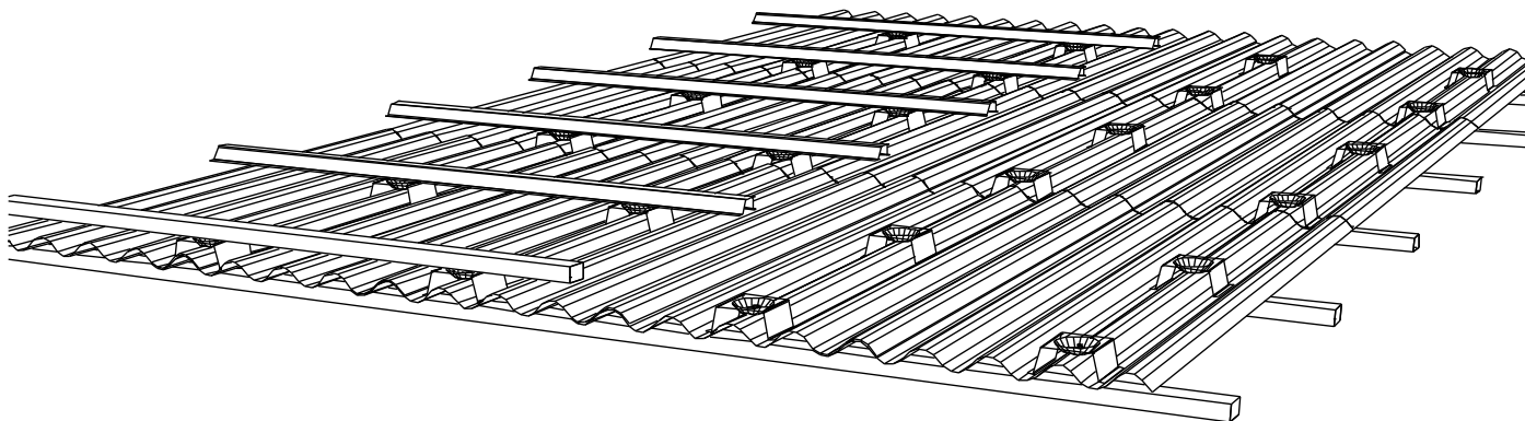
Figur 5.9 Eternittaksrenovering med metod B: Plannja stödbrickor och bärläkt.
