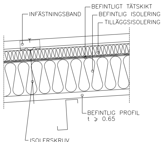
Figur 7.5 Infästningsband mot åsar och bärande plåt längs takfall.
