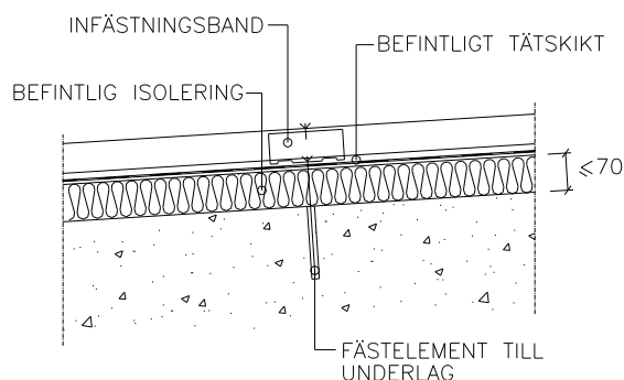
Figur 6.3 Infästning mot isolerad lättbetong eller betong.
