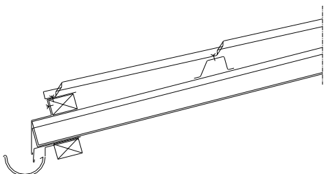
Takfot, befintlig ränna (takpannor)
