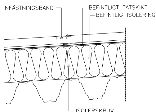
Figur 6.4 Infästning mot bärande plåt tvärs takfall.
