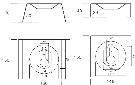
Figur 5.10 Plannja stödbricka för P6 resp. P8.
