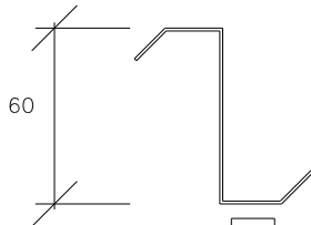
Figur 5.14 Plannja ströläkt för eternitrenovering för P6 och P8.
