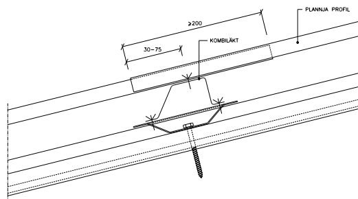
Metod A, stum skarv (profilerad plåt) gäller även metod B
