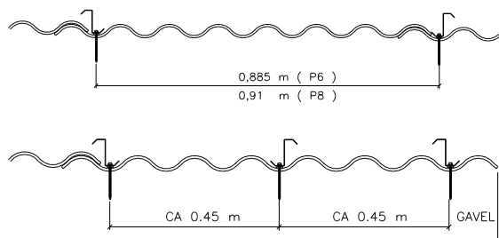
Figur 5.17 Avstånd mellan Plannja ströläkt för eternitrenovering.
