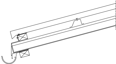
Takfot, ny ränna (profilerad plåt)
