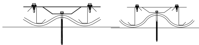
Figur 5.5 Infästning av Plannja stålregel för eternitrenovering till låsbricka på P8 (vänster) och P6 (höger).
