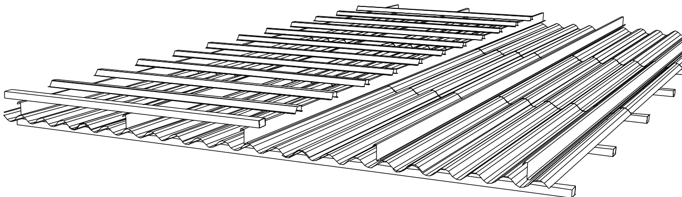
Figur 5.13 Eternittaksrenovering med metod C: Plannja ströläkt/Kombiläkt utan brickor.
