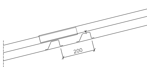
Figur 4.5 Dilatationsskarv.
