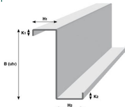
Z-profil
